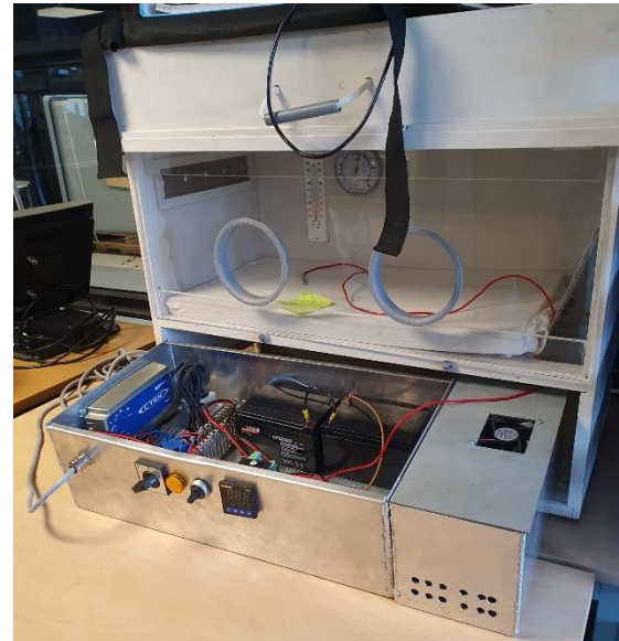
De couveuse geschikt voor Kameroen
